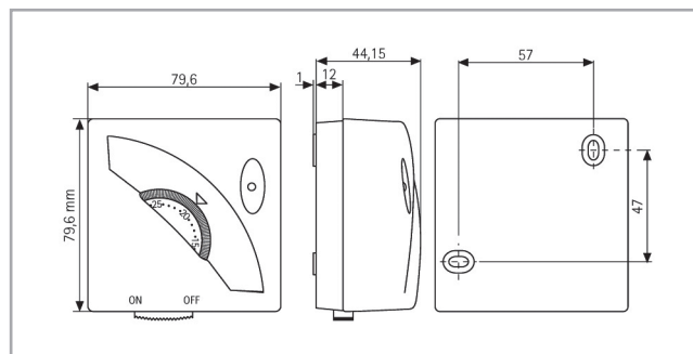
МЕХАНИЧЕСКИЙ КОМНАТНЫЙ ТЕРМОСТАТ
