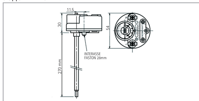
ТЕРМОСТАТ ДЛЯ ЭЛЕКТРИЧЕСКИХ ВОДОНАГРЕВАТЕЛЕЙ
