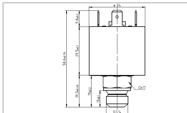
РЕЛЕ ДАВЛЕНИЯ СЕМЕ
